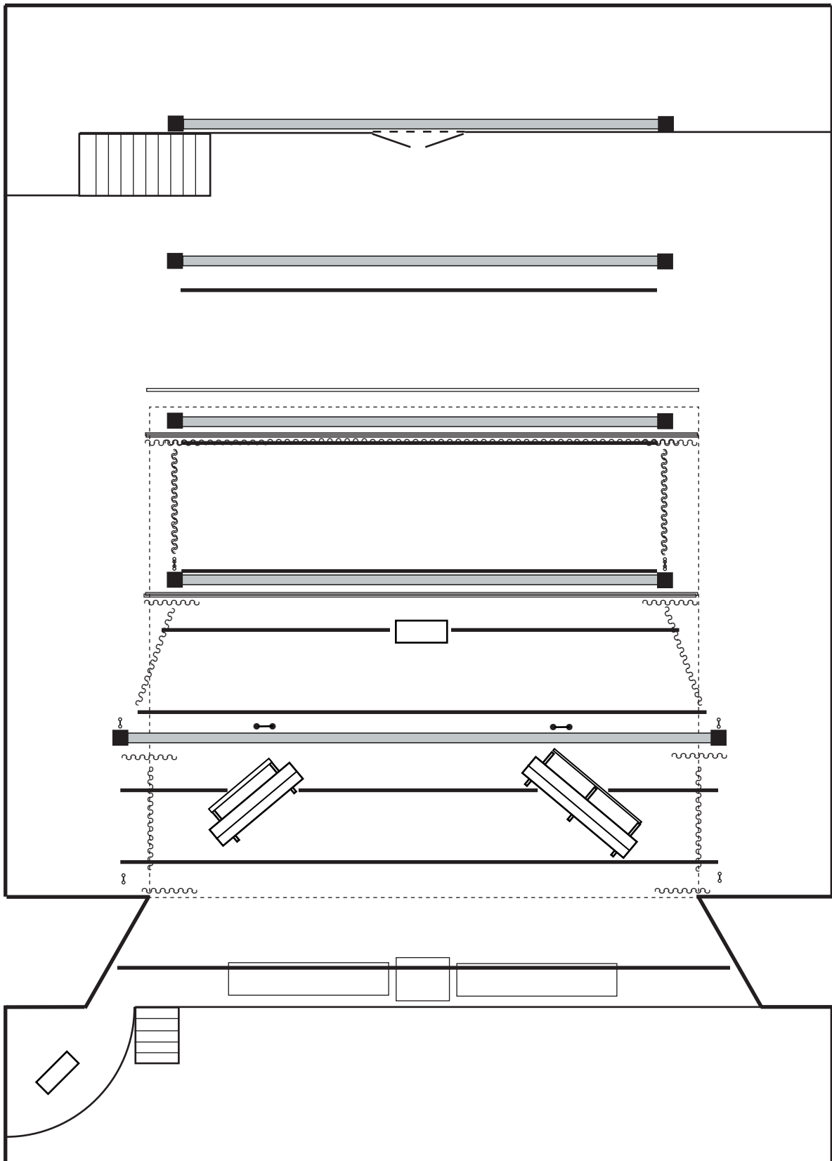
theater Thalia productie DORO bovenaanzicht toneel / decor, afstopping & trekkenplan afmetingen in cm. schaal 1: 100
