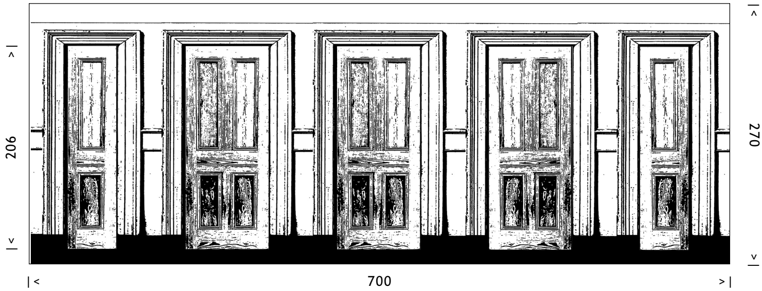
vooraanzicht achtervak mirandolina (maten in cm.)
