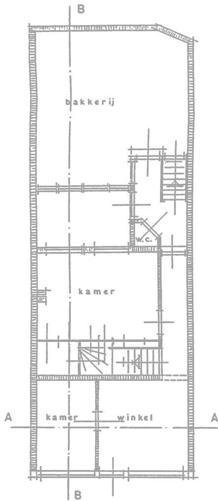
BEGANE GROND
